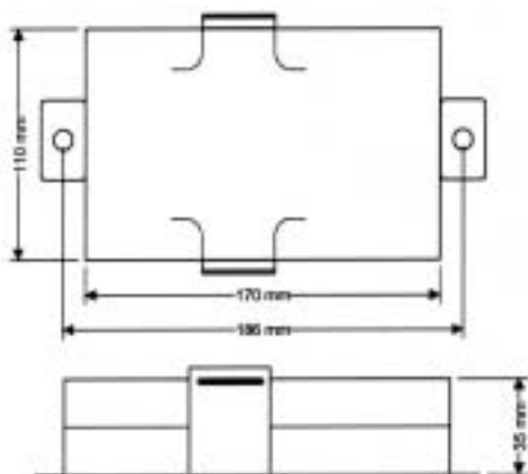
Controller-Gehäuse
